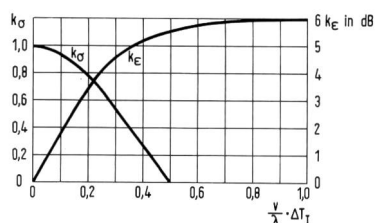
Fig. 3 Korrekturfaktoren für die Feinstrukturstreuung \sigma_F und für den Feldstärkemedianwert \bar{\varepsilon} in Funktion des Weges, der während der Impulsdauer durchfahren wird. (Weglänge in Einheiten der Wellenlänge ausgedrückt)
