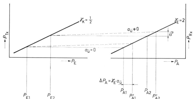
Fig. 6 Übertragungsdämpfung in Kompandern. Ist die Übertragungsdämpfung a_0=0 (horizontale Verbindungslinien), so sind den Eingangspegeln P_{E1} und P_{E2} die Ausgangspegel P_{A1} und P_{A2} zugeordnet. Jede Abweichung der Übertragungsdämpfung von Null ( a_0 \neq 0 ) wird bei der Expansion um den Faktor \gamma_E vergrößert. Atténuation de transmission dans les compresseurs-expandeurs. Si l'atténuation de transmission a_0=0 (lignes horizontales pleines), les niveaux de sortie P_{A1} et P_{A2} sont proportionnels aux niveaux d'entrée P_{E1} et P_{E2} . Chaque déviation de l'atténuation de transmission à partir de zéro ( a_0 \neq 0 ) sera augmentée du facteur \gamma_E lors de l'expansion.
