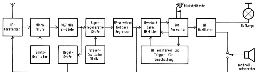
Fig. 3 Prinzipisches Schema des Rufempfängers Schema di principio del ricevitore
