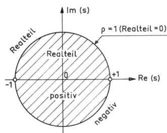
Fig. 4 Lage der Impedanzen in der Ebene des Reflexionsfaktors. Das Innere des Einheitskreises entspricht dem Smith-Diagramm.
