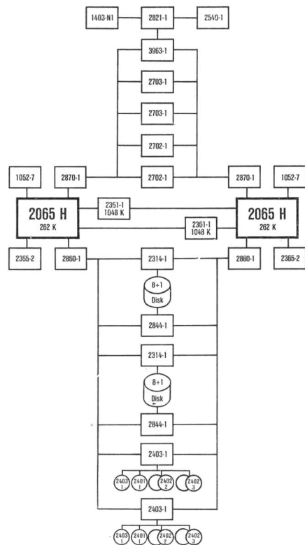
Fig. 8 SWISSAIR Real Time System – Konfiguration Duplex IBM System/360 Modell 65 Ordinateur und unités périphériques du système duplex IBM 360 modèle 65 constituant le système de réservation en temps réel de SWISSAIR
