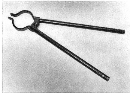
Fig. 1 Spreizzange zum Öffnen und Drehen von Kunststoffrohren (Grösse ca. 75 cm)
