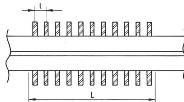
Fig. 9 Abschwächer mit Teilerabstand l und Baulänge L
