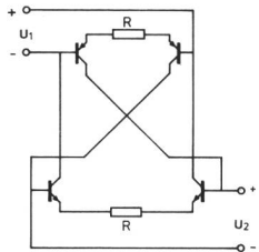
Fig. 3 Prinzipialschaltung eines integrierbaren elektronischen Gyrotors
