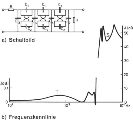
Fig. 4 Telephoniefilter mit Gyrotoren
