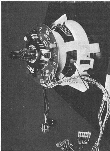
Fig. 1 Die in Amerika entwickelte Dünnhalsröhre mit 110° Strahlablenkung arbeitet mit einer speziellen Ablenkeinheit, mit feineren Elektronenstrahlen und einer von 1,2 auf 1,8 Mio erhöhten Zahl von Leucht-Farbtrippeln. Die Bildgeometrie und die Deckung sollen wesentlich verbessert sein
