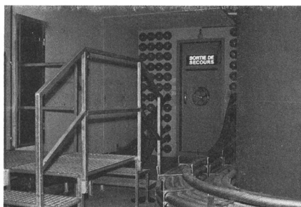
Fig. 2 Une des sorties de secours. On remarque le système étanche de pénétration des câbles
