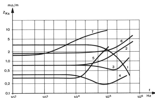
Fig. 3 Kopplungsimpedanz verschiedener Kabelumhüllungen
