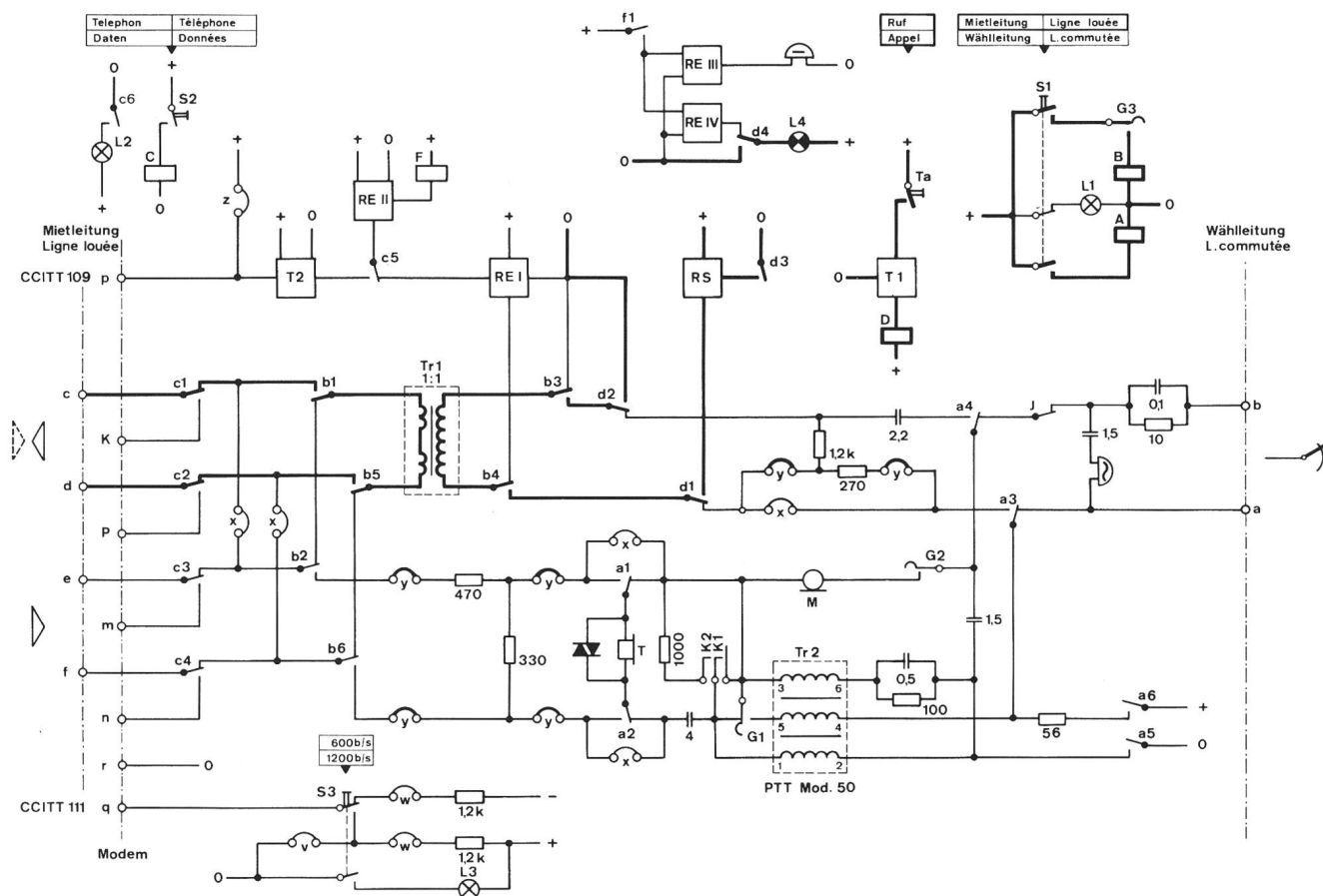
Fig. 6 Stromlaufplan für Ruf auf Mietleitung – Chemin du signal d'appel pour le circuit loué
