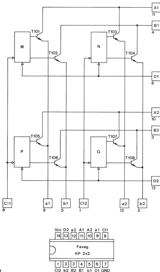
Fig. 8 Blockschema der integrierten Schaltung, mit Bezeichnung der Anschlüsse
