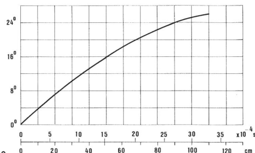
Fig. 10 Einfluss des Zeitunterschieds auf die stereophonische Wahrnehmung
