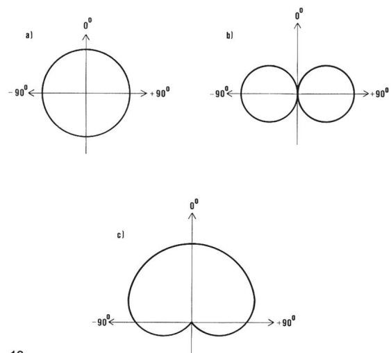
Fig. 12 Mikrofon-Richtcharakteristiken Caractéristiques directionnelles des microphones
