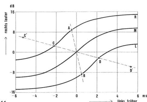
Fig. 11 Einfluss der Kombination aus Intensitäts- und Zeitunterschied auf die stereophonische Wahrnehmung
