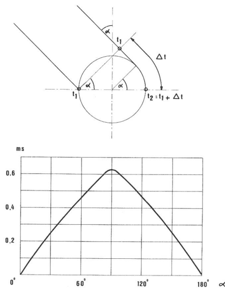
Fig. 5 Laufzeitunterschied als Funktion des Winkels Différence de la durée du parcours en fonction de l'angle
