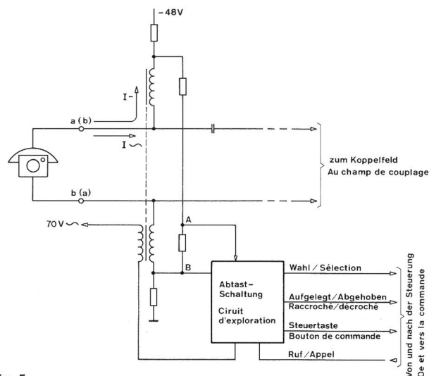
Fig. 5 Prinzip der Teilnehmerschaltung – Principe du circuit d'abonné
