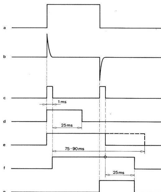
Fig. 5 Diagramm der Impulskontrolle
