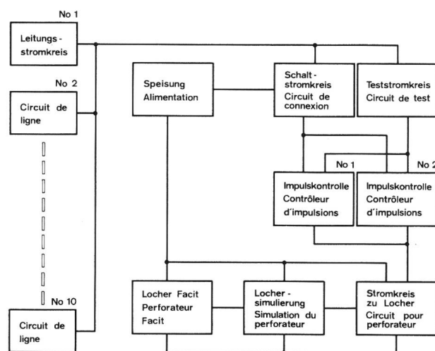
Fig. 3 Blockschema des Zielregistrierungsgerätes
