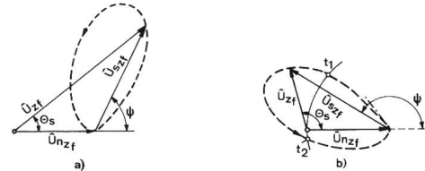
Fig. 4 Zeitlicher Verlauf des Summenvektors
