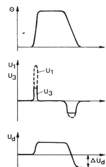
Fig. 8 Spannungssprung bei einem Phasenstoss mit unterschiedlichen Anstiegs- und Abfallzeiten
