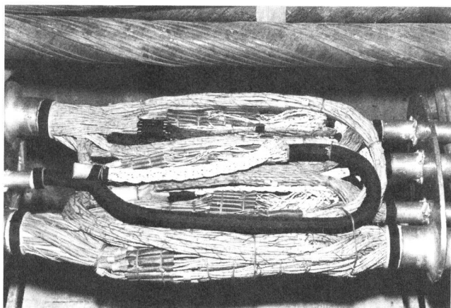
Fig. 14 Innenansicht einer Pupinspleissung – Vue intérieure d'une épissure de pupinisation
