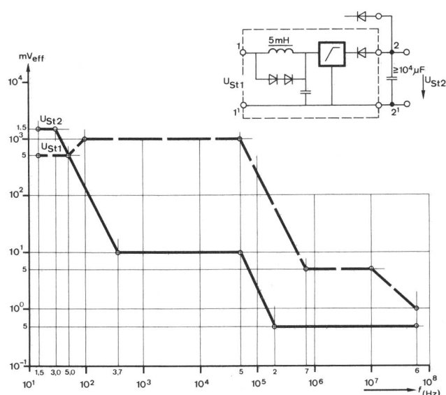
Fig. 4 Zulässige Störspannungen an der Sicherungseinheit – Tensions perturbatrices admissibles au niveau de l'unité de coupe-circuit
