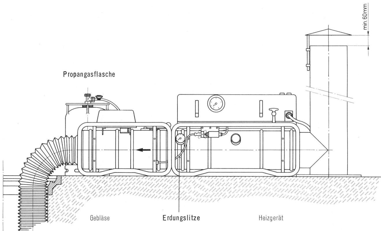
Fig. 3 Betriebsbereite Heizung
