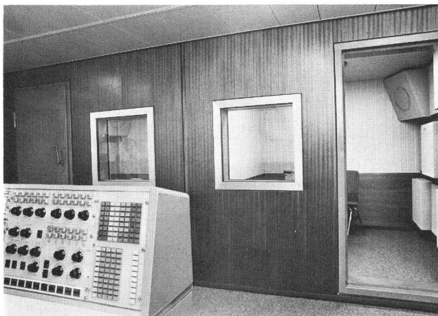
Fig. 2 Ansicht der beiden Kabinen (im Vordergrund Steuerpult) – Vue des deux cabines (au premier plan, le pupitre de commande)
