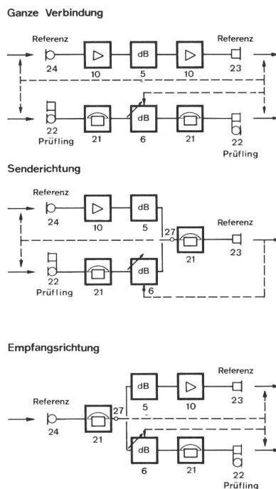
Fig. 8 Blockschema betreffend Lautstärkevergleich zwischen Telefonausrüstung und Referenzsystem – Schéma-bloc concernant la comparaison de volume entre un équipement téléphonique et le système de référence
