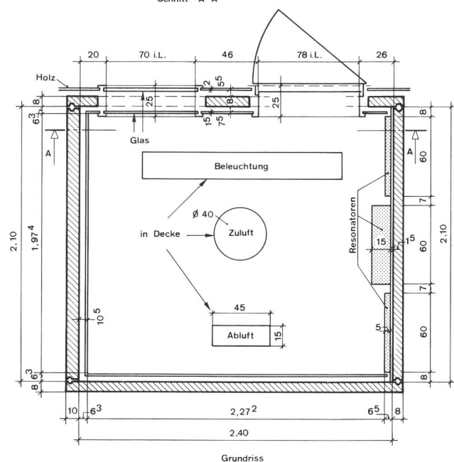
Fig. 4 Abmessungen und Konstruktionsdetails der Kabinen – Dimensions et détails de construction des cabines
