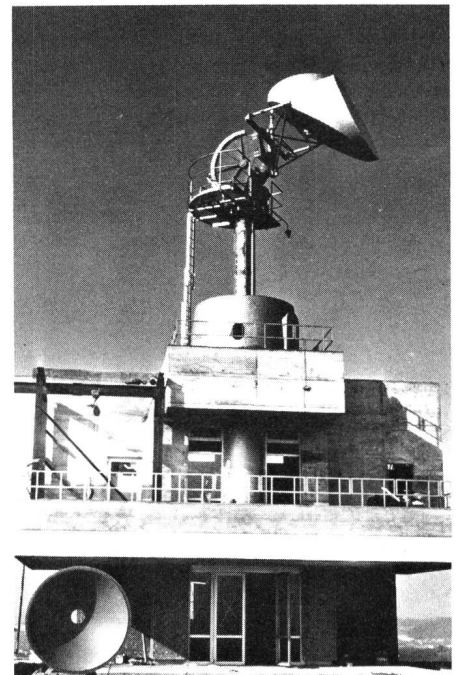
Antennenmessplatz auf dem Dach des Hochhauses der Abteilung Forschung und Entwicklung
