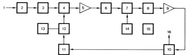
Fig. 6 Empfänger-HF-Kopf
