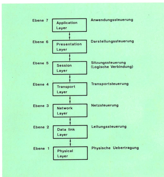
Fig. 9 Sichtenmodell der ISO-Architektur für «offene Systeme» — Modèle des couches de l'architecture ISO pour les «systèmes ouverts» Ebene — Niveau Anwendungssteuerung — Contrôle d'application Darstellungssteuerung — Contrôle de représentation Sitzungssteuerung (logische Verbindung) — Contrôle de séance (liaison logique) Transportsteuerung — Commande du transport Netzsteuerung — Commande du réseau Leitungssteuerung — Commande de liaison Physische Übertragung — Transmission physique
