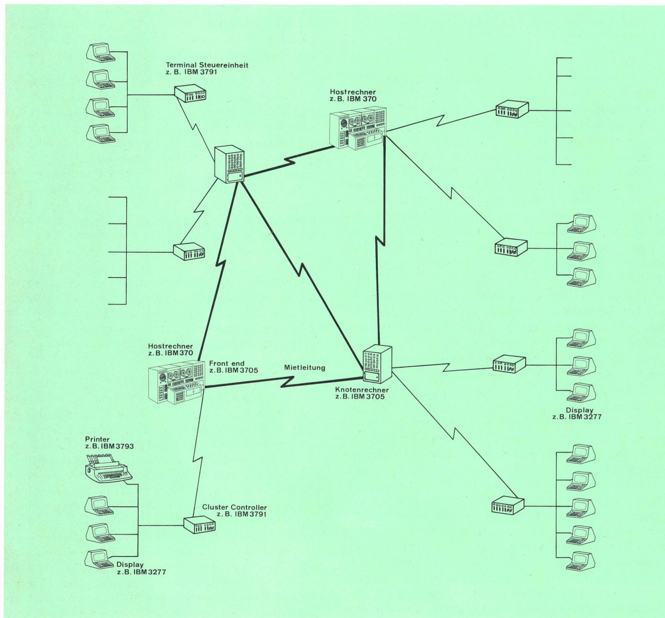
Fig. 2 Privates Datennetz mit Vermittlung, zum Beispiel gemäss Netzarchitektur SNA von IBM — Réseau de données privé avec commutation par exemple selon l'architecture de réseau SNA d'IBM
