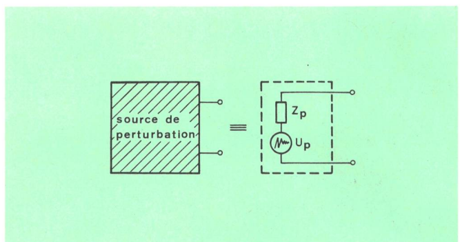
Fig. 4 Source de perturbations équivalente U_p Tension de la source de perturbations Z_p Impédance de la source de perturbations
