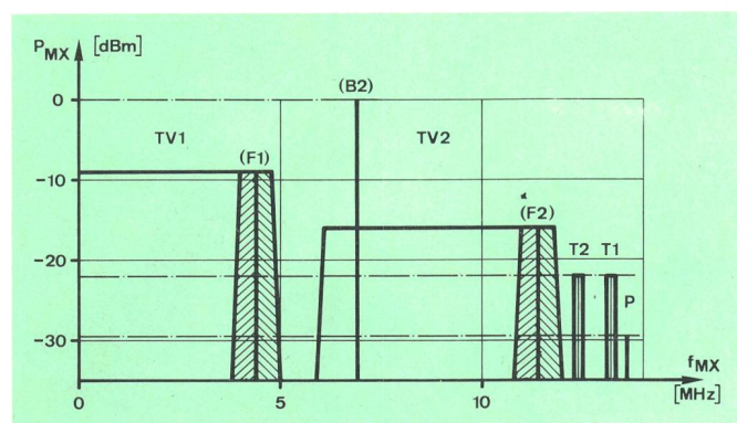
Fig. 3 2-TV-Multiplexsignal, am Pegelpunkt -22 dBr — Signal multiplex 2 TV au point de niveau -22 dBr
