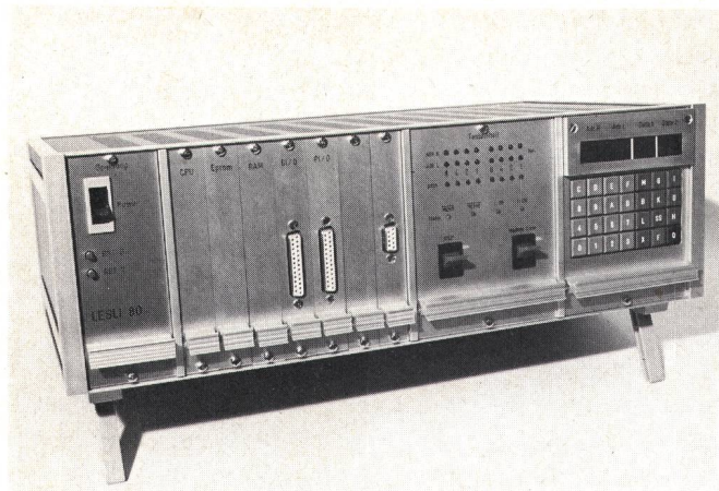
Fig. 7 Mikrocomputer LESLI-80 — Micro-ordinateur d'instruction LESLI-80
