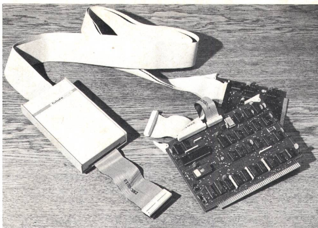
Fig. 4 In-Circuit-Emulator — Emulateur connecté
