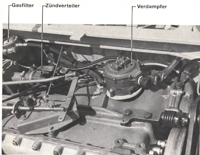
Fig. 7 Saurer-Turbogasmotor 184 kW. Oben rechts der wassergekühlte Verdampfer, links oben ein Gasfilter, darunter der Zündverteiler — Turbomotor zu gas Saurer de 184 kW. En haut à droite le détendeur refroidi à l'eau, à gauche en haut un filtre à gaz, en dessous le distributeur d'allumage
