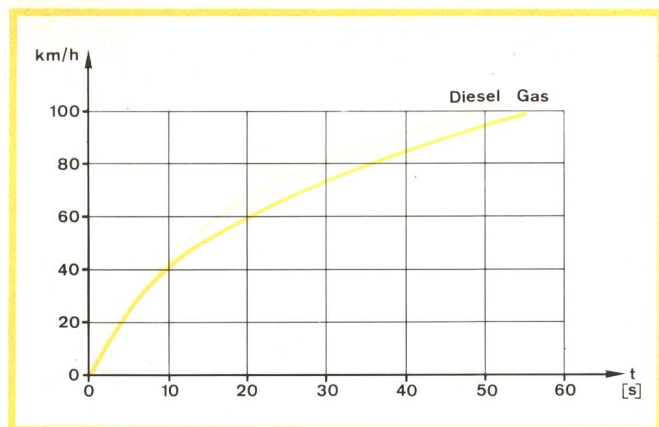
Fig. 10 Beschleunigungszeiten für Busse mit Diesel- und Gasmotor (die Werte gelten für leere Wagen und ebene Strassen) — Temps d'accélération pour bus à moteur diesel et à gaz (les valeurs se rapportent à des voitures vides et des routes plates) Gas — Gaz
