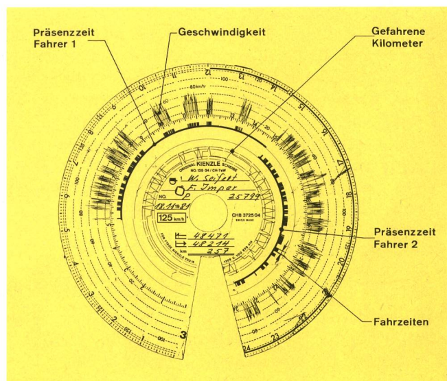
Fig. 12 Fahrtschreiberscheibe eines Kurstages — Disque de tachomètre d'un jour de parcours Präsenzzeit — Temps de présence Fahrer — Chauffeur Geschwindigkeit — Vitesse Gefahrene Kilometer — Kilomètres parcourus Fahrzeiten — Temps de parcours
