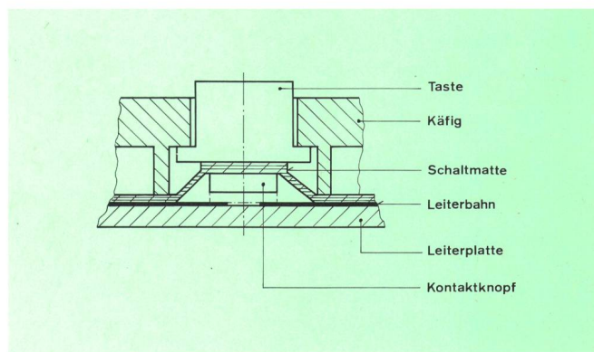
Fig. 3 Querschnitt durch Tastatur — Coupe du clavier Taste — Touche Käfig — Grille Schaltmatte — Membrane de contact Leiterbahn — Plaque conductrice Leiterplatte — Circuit imprimé Kontaktknopf — Bouton de contact
