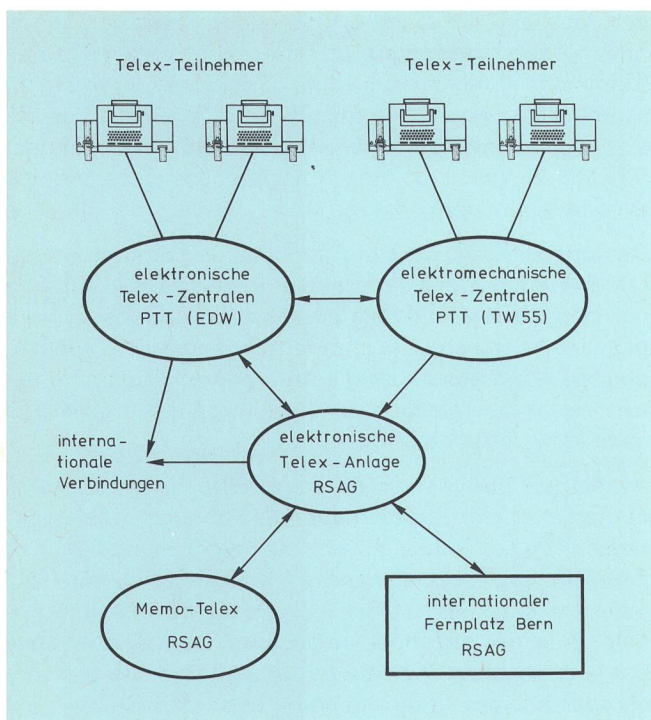
Fig. 1 Das System Memo-Telex im schweizerischen Telex-Netz – Integration des Systems Memo-Telex in das schweizerische Telex-Netz
