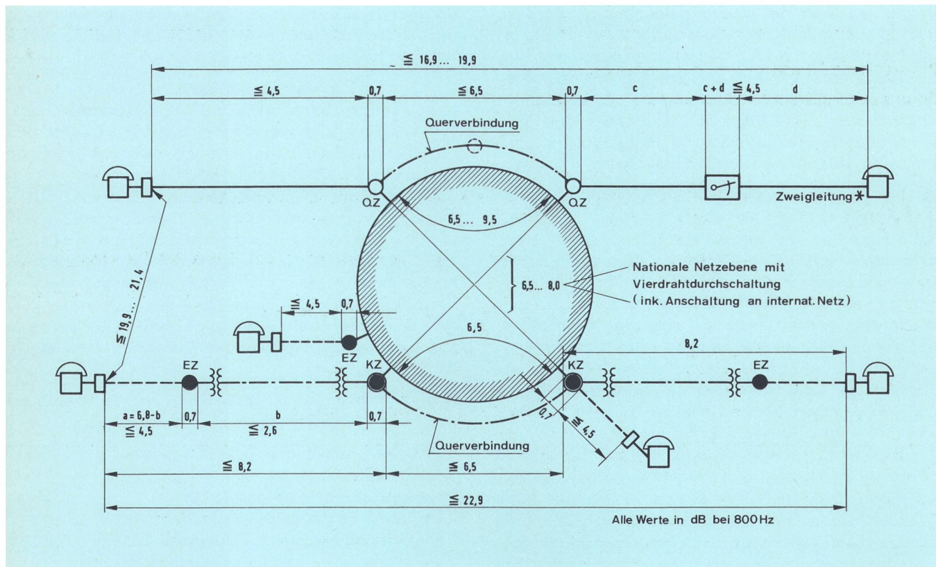
Fig. 2 Dämpfungsplan 1966/1977
