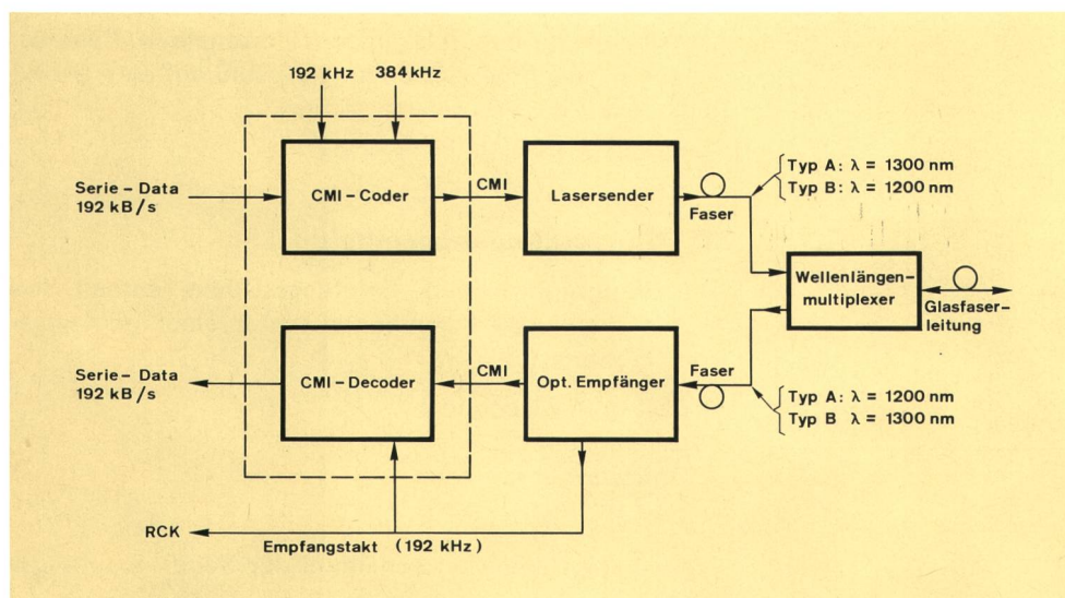
Fig. 4 Blockschema Sende-Empfangseinheit
