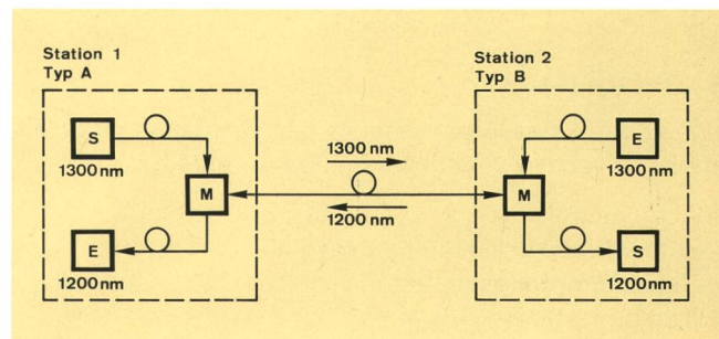
Fig. 1 Bidirektionaler Wellenlängenmultiplex auf einer Glasfaser S Optischer Lasersender E Optischer Empfänger M Wellenlängenmultiplexer — Glasfaserverbindung
