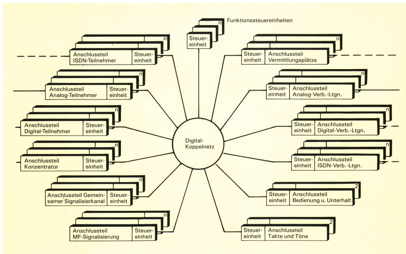
Fig. 1 Modulare Struktur des Systems 12 – Structure modulaire du système 12 Digitalkoppelnetz – Réseau de connexion numérique Funktionssteuereinheiten – Organes de traitement auxiliaire Steuereinheit – Organe de traitement Anschluss-einheit ISDN-Teilnehmer – Terminal d'abonnés RNIS Anschluss-einheit Analog-Teilnehmer – Terminal d'abonnés analogiques Anschluss-einheit Digital-Teilnehmer – Terminal d'abonnés numériques Anschluss-einheit Konzentrator – Terminal d'interface pour concentrateur Anschluss-einheit Gemeinsamer Signalisierkanal – Terminal de canaux sémaphores Anschluss-einheit MF-Signalisierung – Terminal de signalisation multifréquence Anschluss-einheit Vermittlungsplätze – Terminal d'interface d'opératrice Anschluss-einheit Analog-Verbindungsleitungen – Terminal de jonctions analogiques Anschluss-einheit Digital-Verbindungsleitungen – Terminal de jonctions numériques Anschluss-einheit ISDN-Verbindungsleitungen – Terminal de jonctions RNIS Anschluss-einheit Bedienung und Unterhalt – Terminal de maintenance et périphériques Anschluss-einheit Takte und Töne – Unité d'horloge et de tonalités
