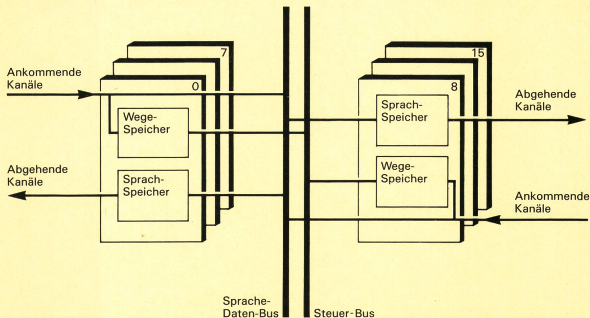
Fig. 2 Prinzip der Koppelbaugruppe mit 16 Ports – Principe de la carte de commutation numérique Ankommende Kanäle – Canaux entrants Wege-Speicher – Mémoire d'itinéraire Abgehende Kanäle – Canaux sortants Sprach-Speicher – Mémoire de parole Sprach-/Daten-Bus – Bus pour voix et données Steuer-Bus – Bus de commande
