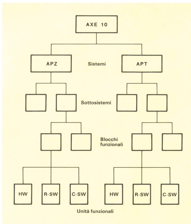
Fig. 2 Struttura del sistema AXE 10 APT Sistema di commutazione APZ Sistema di comando HW Hardware
