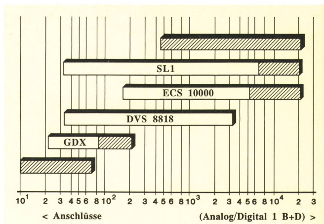
Fig. 32 PTT-Angebot digitale TVA – Offres des PTT en ECA numériques Anschlüsse – Raccordements (analog/digital 1B + D) – (analogique/numérique 1B + D)
