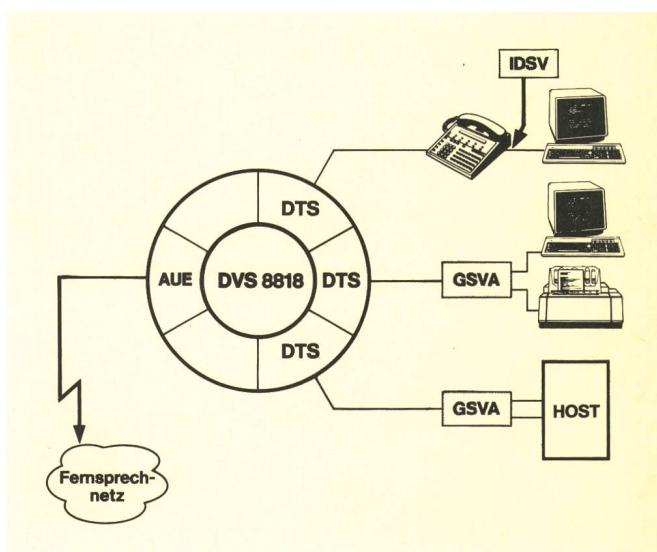
Fig. 14 DVS-8818-Datenkommunikation (Beispiel) – Communication de données DVS 8818 (exemple) Fernsprechnetz – Réseau téléphonique
