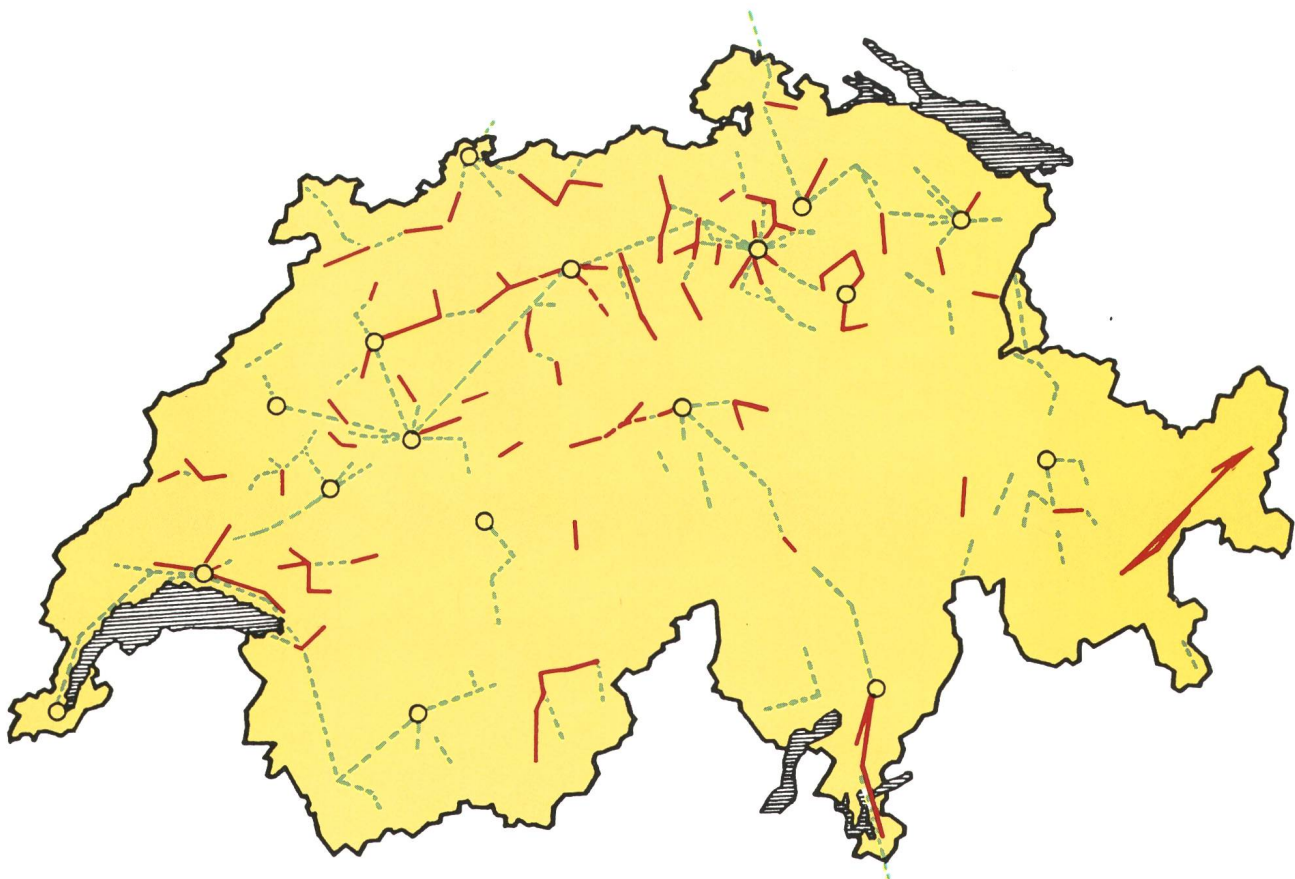
Fig. 4 Kabelanlagen mit Glasfasern Impianti di cavi in fibra ottica — Anlagen 1984–1990 — Anlagen 1991–1995 Impianti 1984–1990 Impianti 1991–1995
