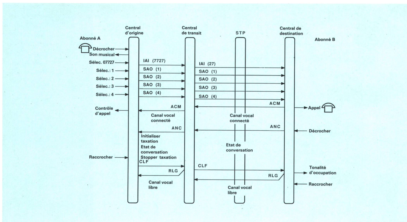
Fig. 16 Etablissement et déconnexion d'une communication avec TUP (raccordements d'abonnés analogiques) – Formazione e scioglimento della comunicazione con TUP (collegamenti di tipo analogico)
