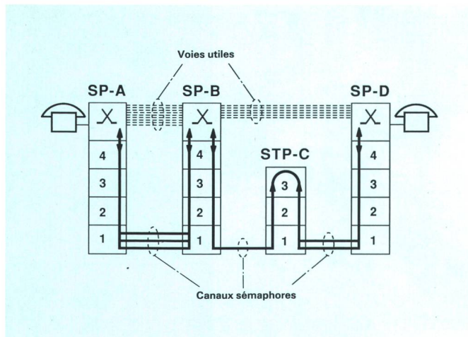
Fig. 4 Réseau de la figure 3 selon la structure des niveaux – Rete di figura 3 nella struttura a livelli Voies utiles – Canali utili Canaux sémaphores – Canali di segnalazione
