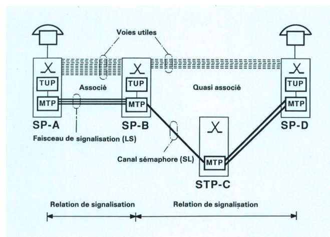
Fig. 3 Structure du réseau et composants – Struttura e componenti della rete
