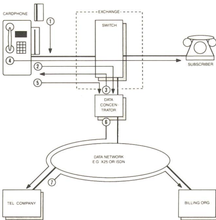
Déroulement général du traitement des données lors d'une communication téléphonique avec carte de crédit.
