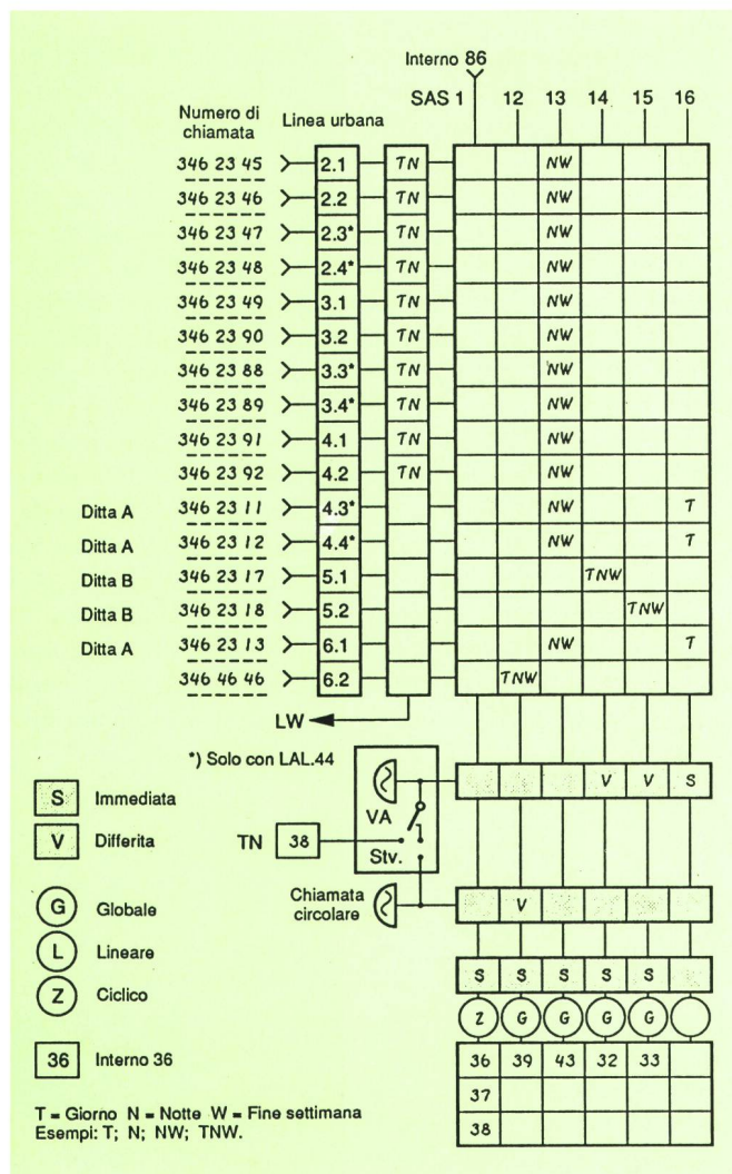
Fig. 6 Il foglio relativo alla distribuzione delle chiamate fornisce chiare informazioni sui sei fasci dei collegamenti collettivi programmati per la ditta
