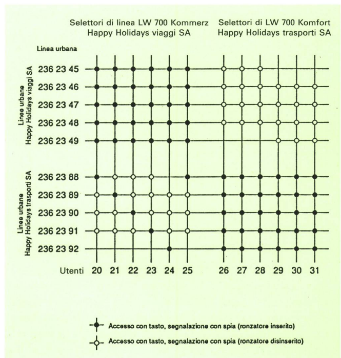
Fig. 5 Accesso alle linee con i selettori di linea LW 700 nell'ufficio viaggi e nella divisione trasporti
