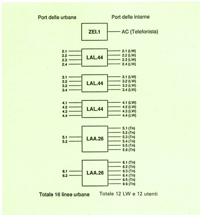
Fig. 2 Configurazione dell'ICU ibrido della ditta Happy Holidays: L'impianto richiede un contenitore equipaggiato completamente
