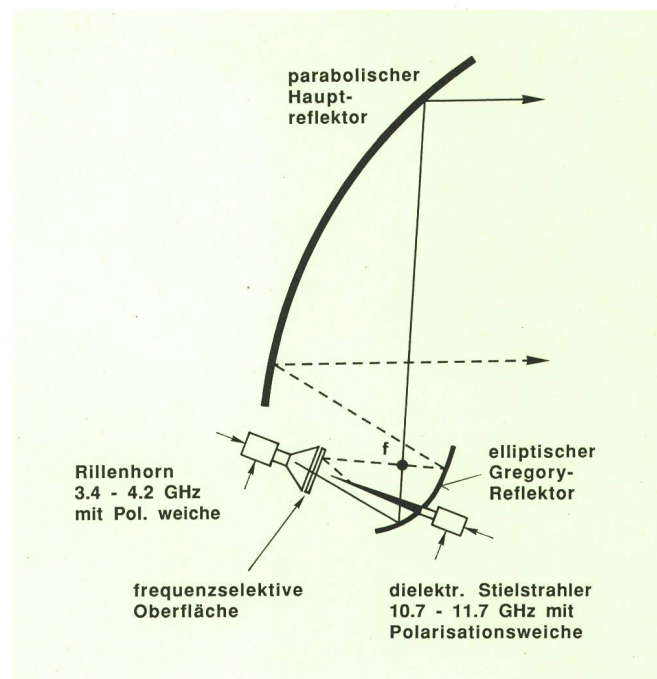
Fig. 6 Prinzip der XPD-optimierten Dualband-Offsetantenne für 4 und 11 GHz – Principe de l'antenne à source primaire décalée pour 4 et 11 GHz, optimisée en ce qui concerne les valeurs de découplage XPD
