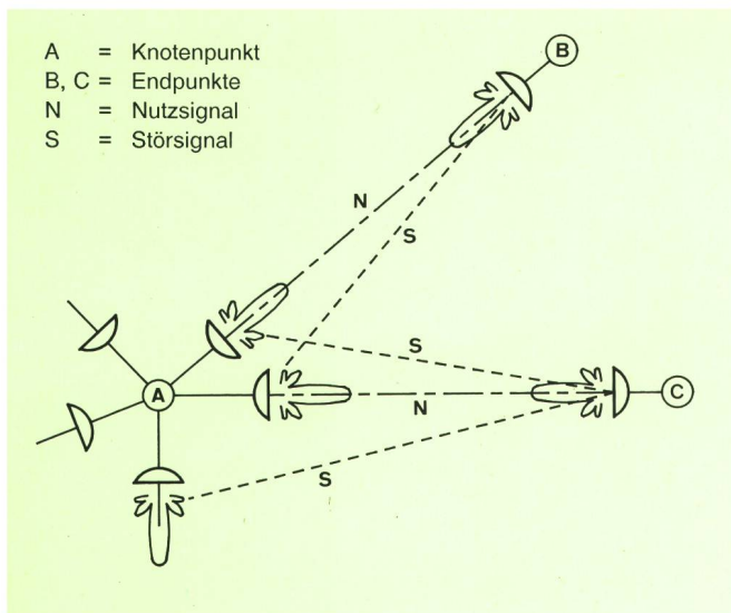
Fig. 2 Entstehung von Gleichkanalstörungen auf Richtfunk-Knotenpunkten – Apparition de perturbations sur le même canal dans les nœuds de transmission par faisceaux hertziens
