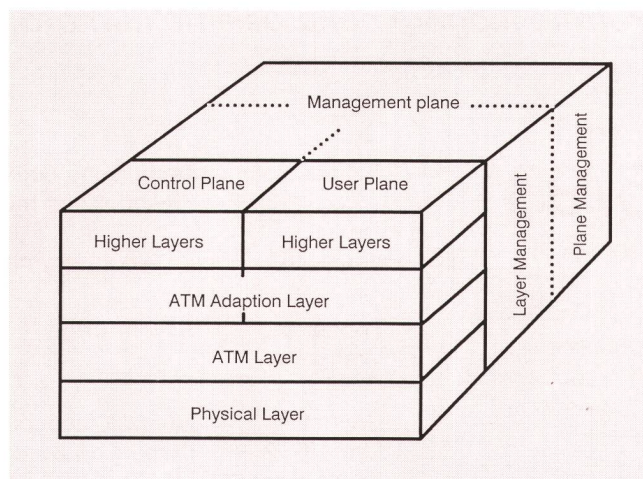
Fig. 1 B-ISDN-Protokoll-Referenzmodell
