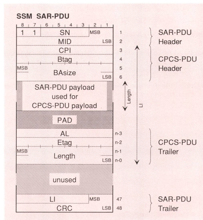
Fig. 5 Ein-Zellen-CPCS-PDU
