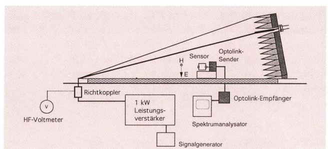
Fig. 7 Messaufbau in der GTEM-Zelle
