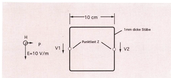
Fig. 5 Modell für die numerische Simulation: Vier ideal leitende Stäbe bilden eine Schleife
