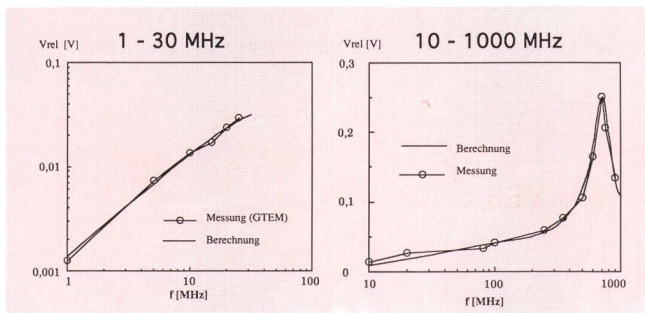
Fig. 8 Vergleich zwischen Messung und Berechnung für zwei Frequenzbereiche: 1 bis 30 MHz und 10 bis 1000 MHz
