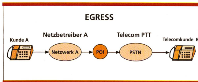
Bild 1. Die Telecom PTT terminiert den Verkehr des Netzbetreibers A zu seinem Telecom-Kunden B. POI: Point of Interconnection (z. B. Eingang oder Ausgang der Transitzentrale); Netzbetreiber: Drittfirma, die eine Konzession für den Betrieb eines Netzes besitzt; Netzwerk: eigenes oder mit Mieteleitungen aufgebautes Netzwerk, das die Vermittlung und Übertragung von Informationen ermöglicht; Kunde A, B: Endkunde, der ein Endgerät in Form eines Telefon-, Fax- oder Datenübertragungsgerätes betreibt.
