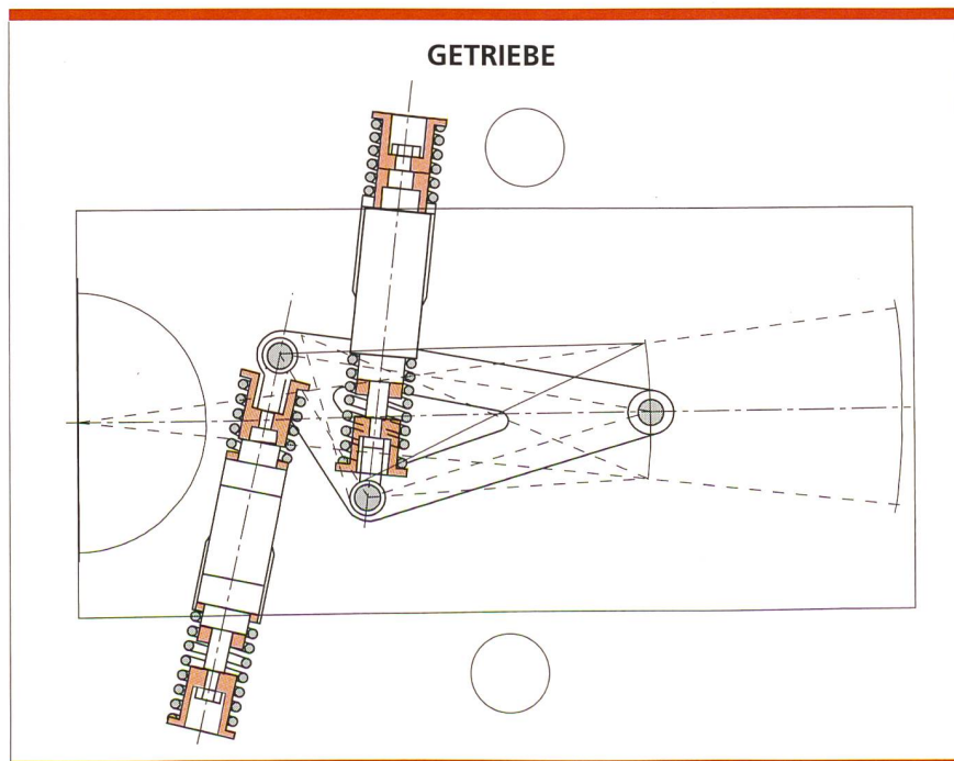
Bild 3. Dreipunkt-Schwenkgetriebe.
