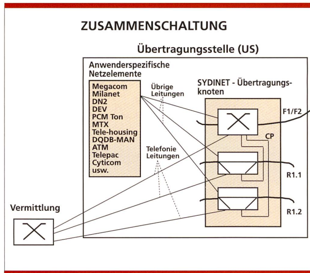
Bild 13. Verbindungen zwischen den Vermittlungseinheiten und den anwenderspezifischen Netzelementen zum SDH-Netzknotten in einer Übertragungsstelle.
