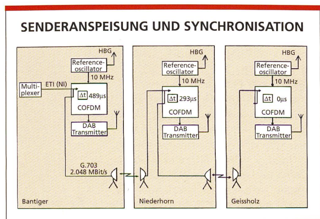
Bild 13. Sende- anspeisung und Synchronisation, Frequenzblock 12B.
