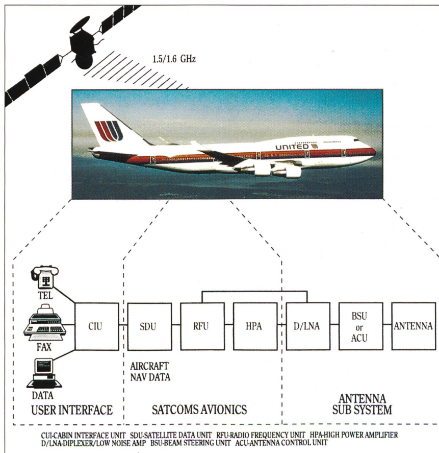
Bild 5. AES-Bordstation.
