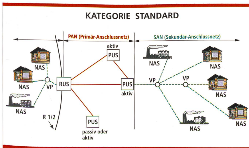
Bild 4. Anschlussnetzkatgorie Standard.
