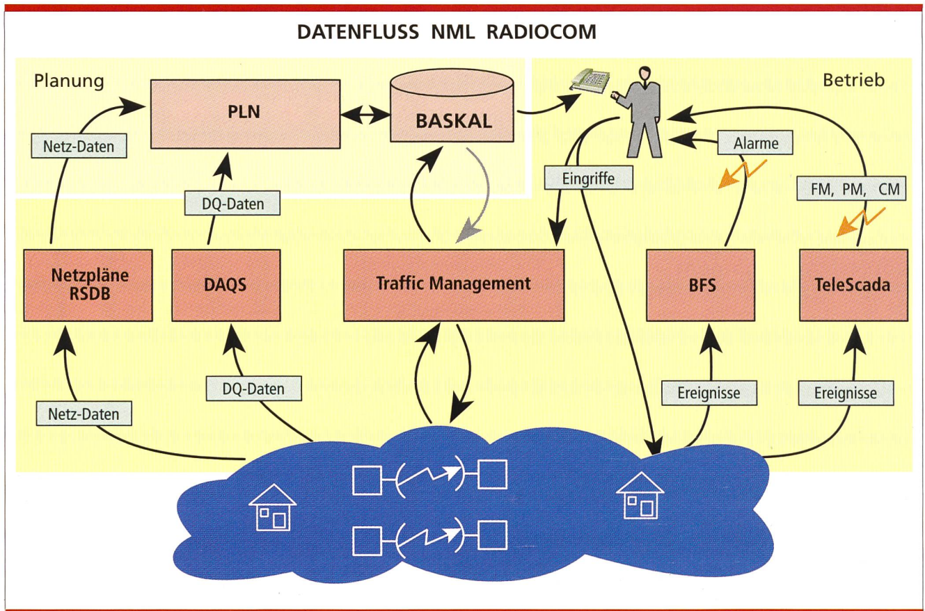
Bild 5. Datenfluss NML Radiocom. RSDB: Datenbank für die Richtstrahlverbindungen. BFS: erfasst Alarme und Betriebszustände; ermittelt zusätzlich die Dienstqualität und generiert statistische Auswertungen. DAQS: ermittelt die Dienstqualität und generiert grafische Auswertungen. TeleScada: erfasst SDH-Richtfunkalarne bei Radiocom. RSDB: Richtstrahl-datenbank; BFS: Betriebsführungssystem; DAQS: Data Acquisition and Quality Supervision; Tele Scada: Netzmanagementplattform der Firma NERA; PLN: Planungssystem Netze; BASKAL: Bewirtschaftungssystem für Systeme, Kabel und Leitungen.
