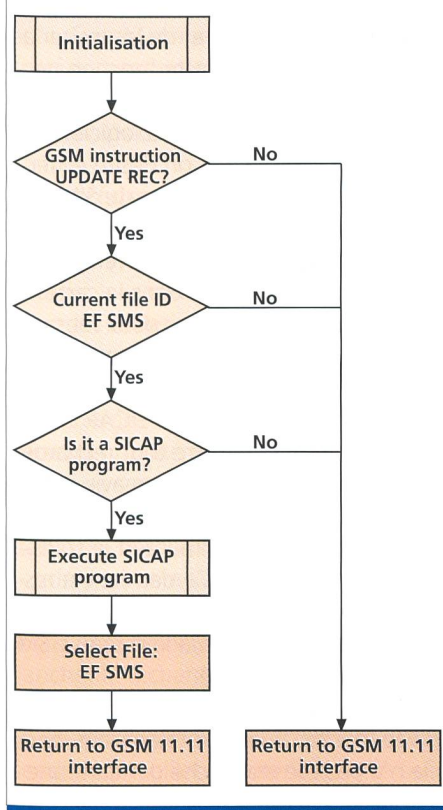
Fig. 2. Mécanisme de filtrage réalisé sur la carte SIM.
