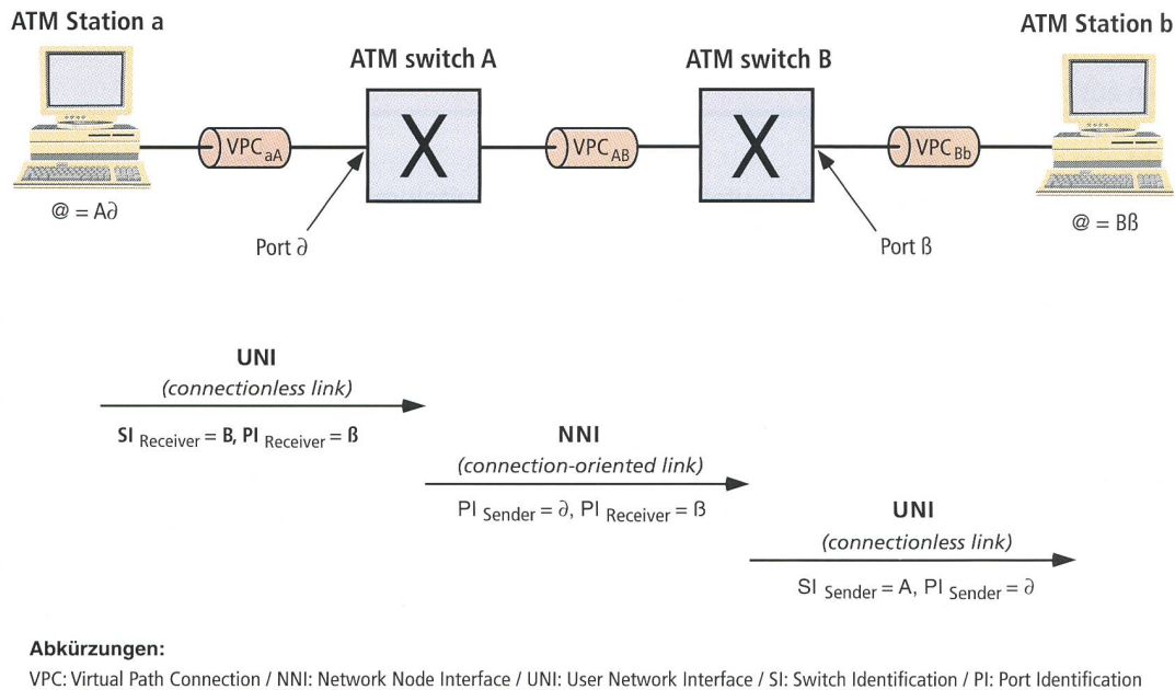
Bild 2. Verbindung zweier ATM-Stationen über Kurzadressen. VPC: Virtual Path Connection, NNI: Network Node Interface, UNI: User Network Interface, SI: Switch Identification, PI: Port Identification.
